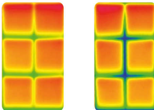
30 pav. Kairėje – šalčio tiltas esant „šiltam“ sudalinimui, dešinėje – naudojant aliumininį sudalinimą
