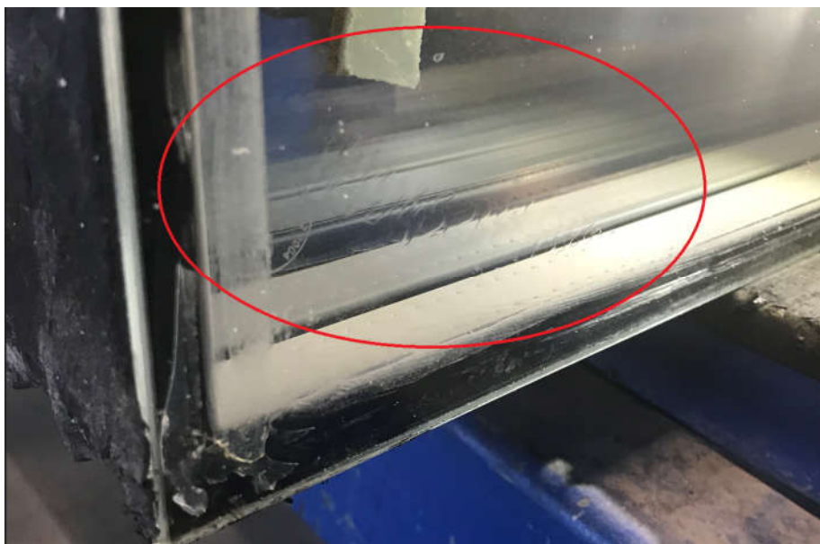
32 pav. PVB plėvelės išsilaminavimas dėl cheminio nesuderinamumo
