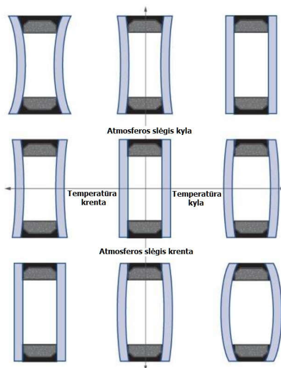
25 pav. Stiklų įsigaubimas/išsigaubimas priklausomai nuo temperatūros ir atmosferos slėgio
