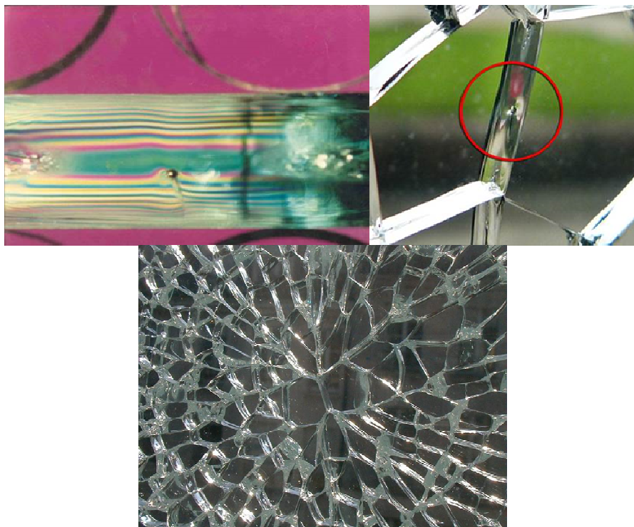
35 pav. Spontaniškos stiklo skilimo pradžia
