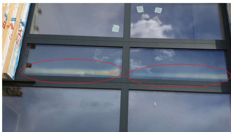
33 pav. Cheminis garavimas stiklo paketo viduje, viršijus rekomenduojamą 60 °C temperatūrą
