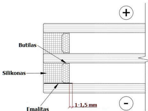
24 pav. Emaliavimo zona struktūriniam stiklinimui skirtiems stiklo paketams
