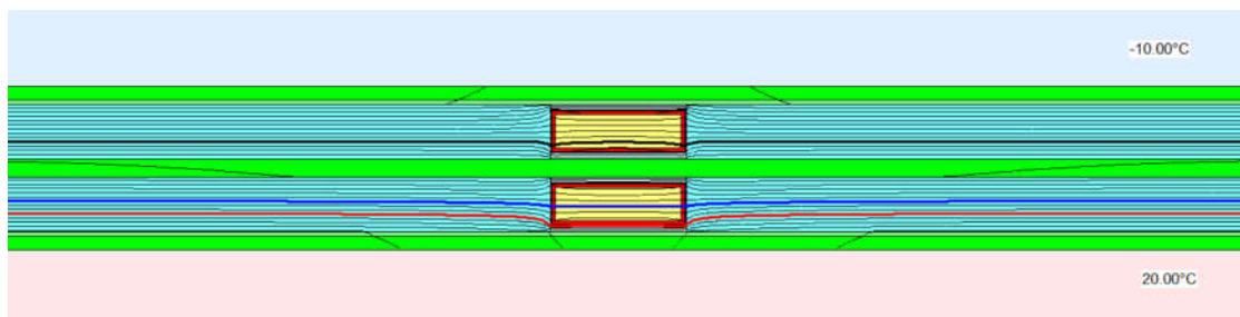
29 pav. Linijinis šiluminis pralaidumas, kai minimali paviršiaus temperatūra -10^\circ \text{C} išorėje (juoda 0^\circ \text{C} , mėlyna 10^\circ \text{C} , raudona 13^\circ \text{C} izoterminė linija)
