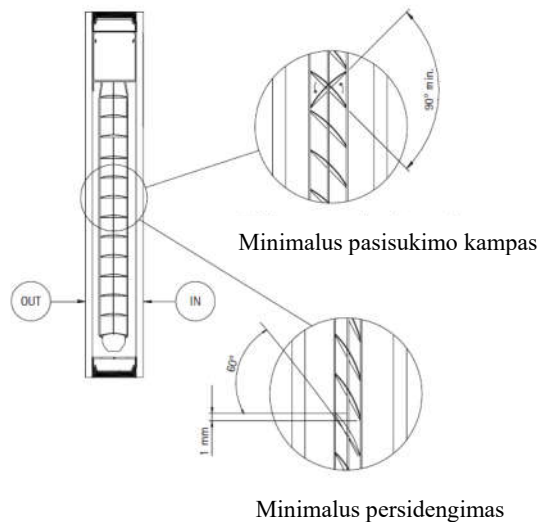
18 pav. Juostelių persidengimas
