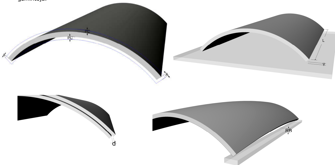
19 pav. Lenktų stiklų nuokrypis
