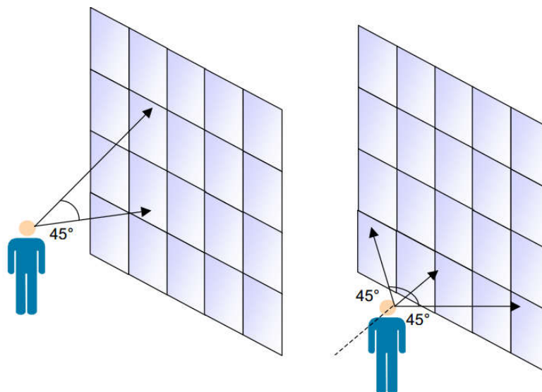
28 pav. Galimas maksimalus kampas vertinant atspalvių skirtumus objekte
