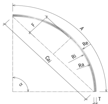
Fig. 23 Parameter of bended glass pane
