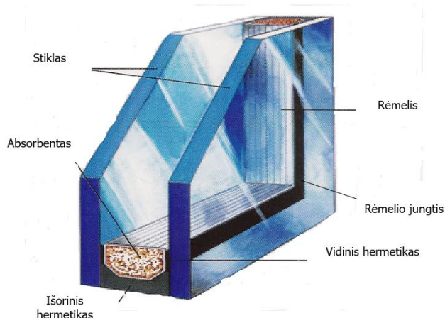
1 pav. Standartinė vienkamerinio stiklo paketo struktūra
