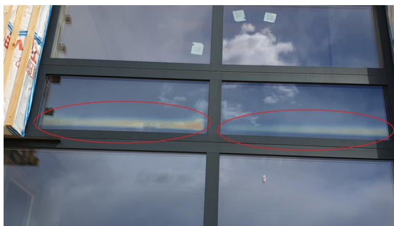
36 pav. Cheminis garavimas stiklo paketo viduje, viršijus rekomenduojamą 60 °C temperatūrą
