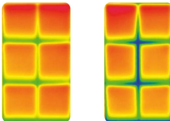
33 pav. Kairėje – šalčio tiltas esant „šiltam“ sudalinimui, dešinėje – naudojant aliumininį sudalinimą
