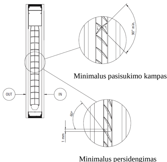
21 pav. Juostelių persidengimas
