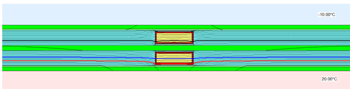
32 pav. Linijinis šiluminis pralaidumas, kai minimali paviršiaus temperatūra -10^\circ\text{C} išorėje (juoda 0^\circ\text{C} , mėlyna 10^\circ\text{C} , raudona 13^\circ\text{C} izoterminė linija)
