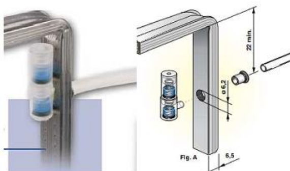
12 pav. Slėgio vožtuvo montavimas į stiklo paketą
