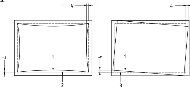
8 pav. Galimi rėmelio netolygumo variantai (1 – rėmelis, 2,3 – teorinė rėmelio priklijavimo pozicija ir forma, 4 – deviacija)
