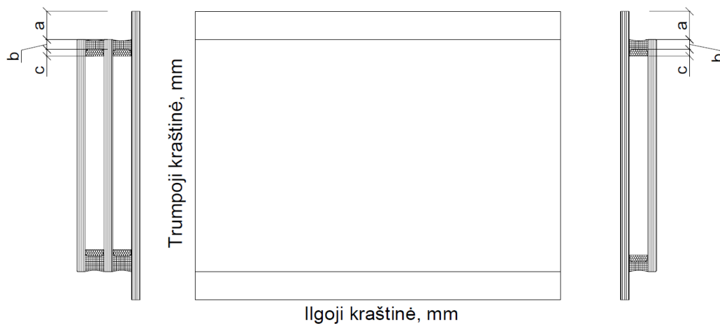
3 pav. Struktūrinio stiklo paketo brėžinys
